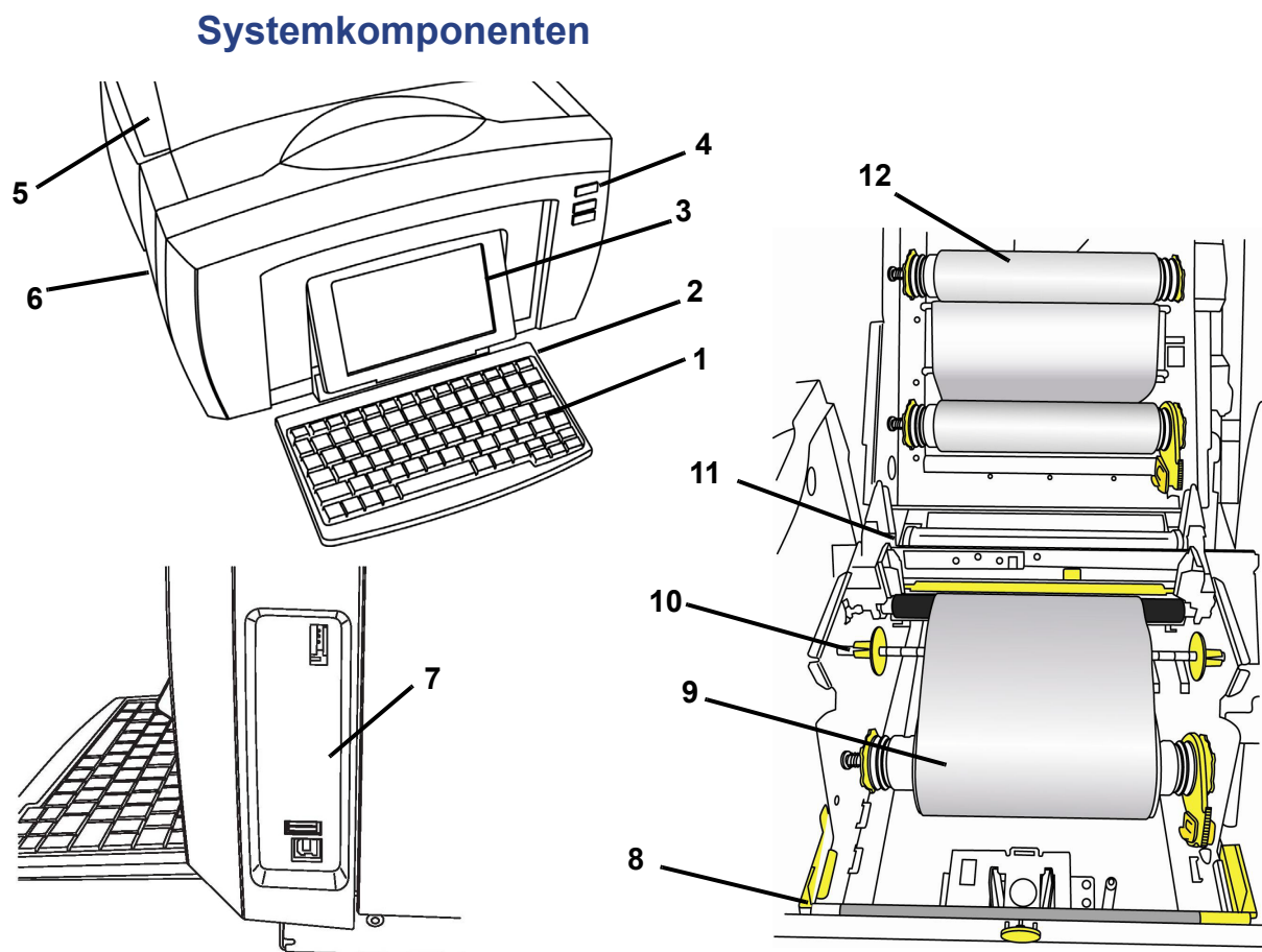
Abbildung 2-1. Druckerkomponenten
